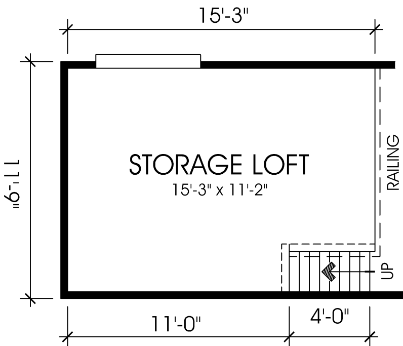
OPTIONAL LOFT AREA
